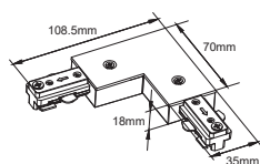
L-Feed-L-3 wires
