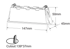
DL694005
