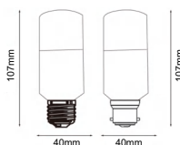
LED-A40-9W
